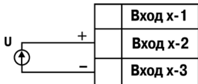
Рисунок Б.7 – Схема подключения активного датчика с выходом в виде напряжения -50\dots 50 мВ или 0\dots 1 В
