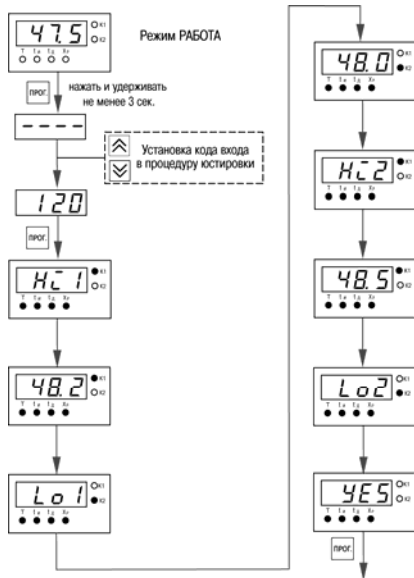
Рисунок Е.2 – Последовательность запуска и индикации АНР для TRM12-Щ1.P
