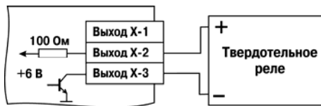
Рисунок Б.4 – Схема подключения нагрузки к ВУ типа Т
