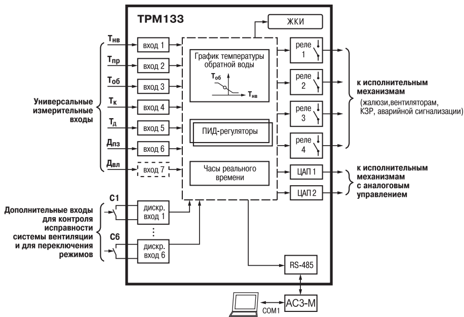
Рис. 3.2. Структурная схема прибора
