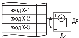
в) датчик с унифицированным выходным сигналом тока
