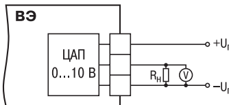
Рис. И.2. Схема подключения пассивного ВЭ типа «ЦАП 0...10 В»
