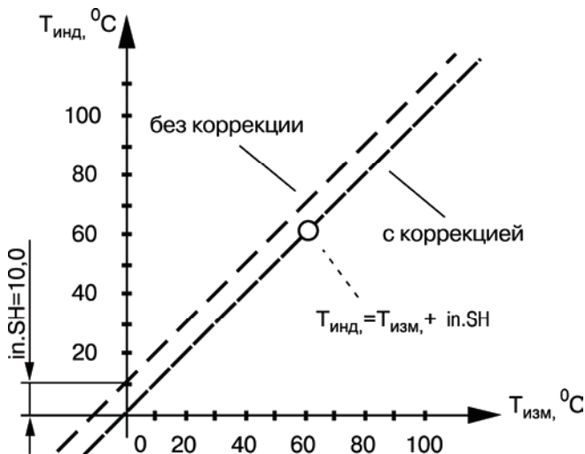
Рисунок 3.6 – Коррекция «сдвиг характеристики»
