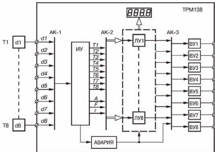
Рисунок 3.1 – Функциональная схема прибора
