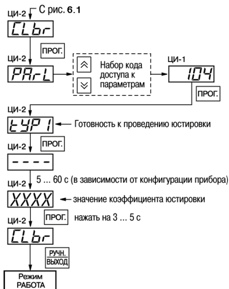
Рисунок Д.2 – Схема проведения юстировки прибора для работы с первичным ЫЗпреобразователем
