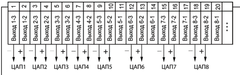
Рисунок Б.5 – Схема подключения ЦАП прибора ТРМ 138-И: а) в корпусе Щ4, б) в корпусе Щ7
