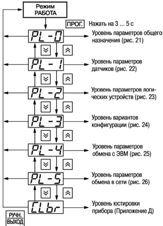
Рисунок 6.1 – Схема выбора уровня программируемых параметров
