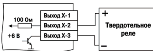
Рисунок 3.18 – Использование транзисторного ключа для управления твердотельным реле
