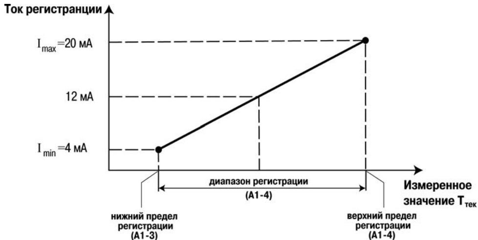
Рисунок 3.14 – Принцип формирования тока регистрации
