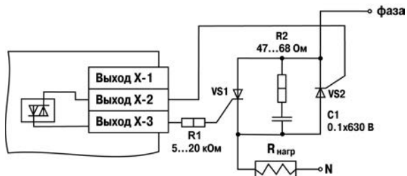
Рисунок Б.4 – Схема подключения к ВУ типа С двух тириستоров, подключенных встречно-параллельно
