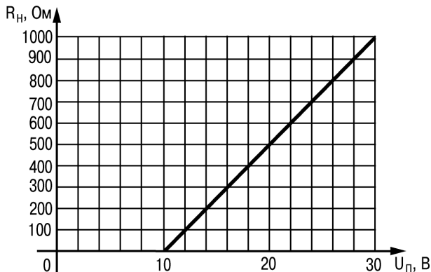
Рисунок 3.16 – График зависимости R_n ( U_n )
