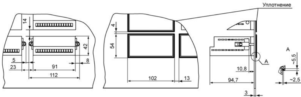
Рисунок А.6 - Прибор в корпусе Щ2, установленный в щит толщиной 3 мм
