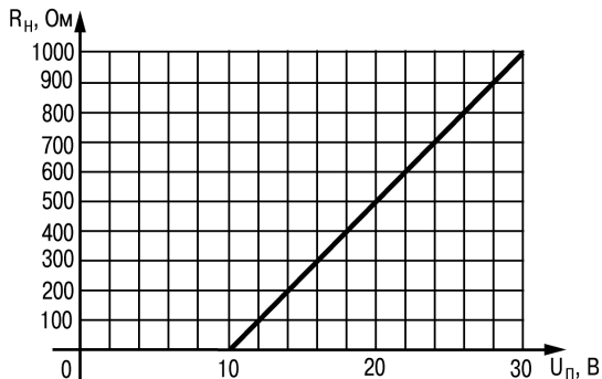
Рисунок 3.16 – График зависимости R_H(U_H)
