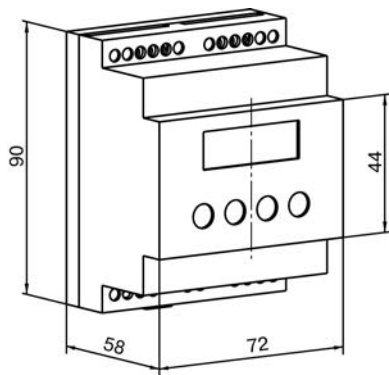
Рисунок А.4 - Прибор с креплением на DIN-рейку Д
