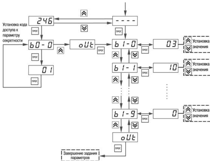
Рисунок 6.3 – Последовательность работы с прибором на втором уровне программирования (для группы параметров b)
