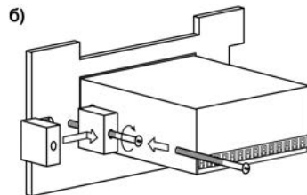
Рисунок 5.2 - Монтаж прибора щитового крепления
