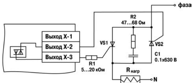
Рисунок Б.4 – Схема подключения к ВУ типа С двух тириستоров, включенных встречно-параллельно
