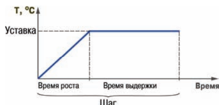
Рис. 3.12. Схема шага Программы технолога
