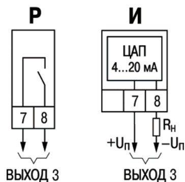
Рис. Б.4. Схемы подключения к различным типам Выходного элемента 3
