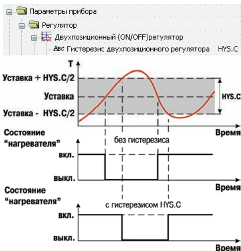
Рис.3.4. Принцип работы двухпозиционного регулятора
