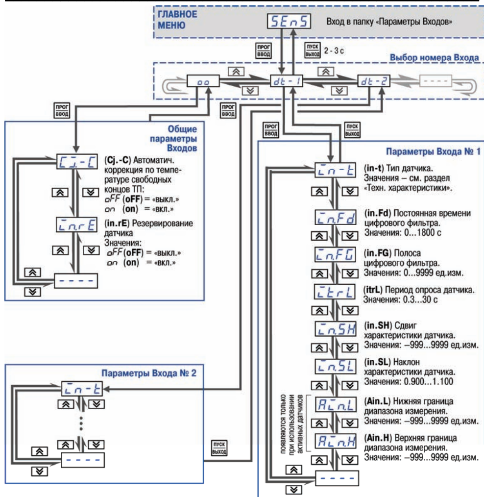
Рис. 7.5. Схема задания параметров Входов
