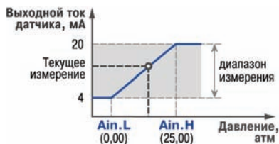
Рис.3.2. Пример задания диапазона измерения
