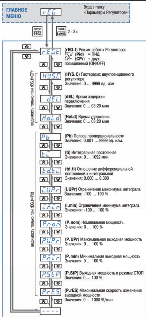
Рис. 7.2. Схема задания параметров Регулятора
