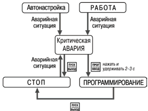
Рис. 8.2. Схема переключения режимов при Критической АВАРИИ
