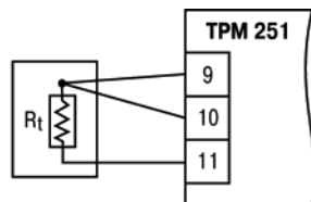
Рис. Г.1. Схема подключения ТС по трёхпроводной схеме
