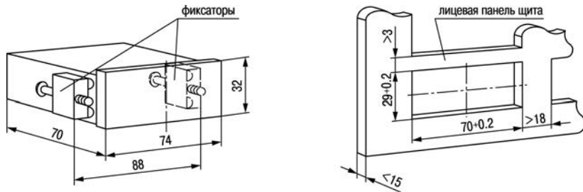
Рисунок А.1 – Габаритные и установочные размеры TPM501
