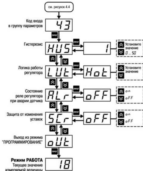
Рисунок 4.8 – Схема установки параметров регулятора
