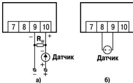
Рисунок 6.4 – Схема подключения датчиков с выходным сигналом тока (а) и напряжения (б)
