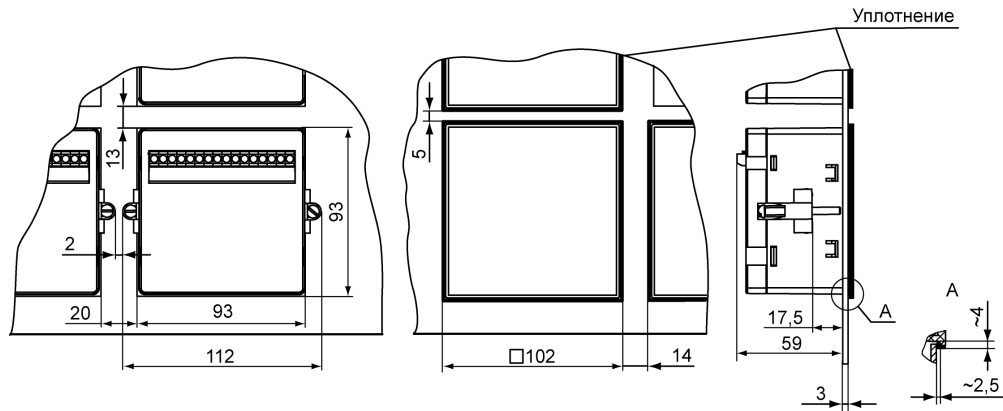
Рисунок А.6 - Прибор в корпусе Щ1, установленный в щит толщиной 3 мм
