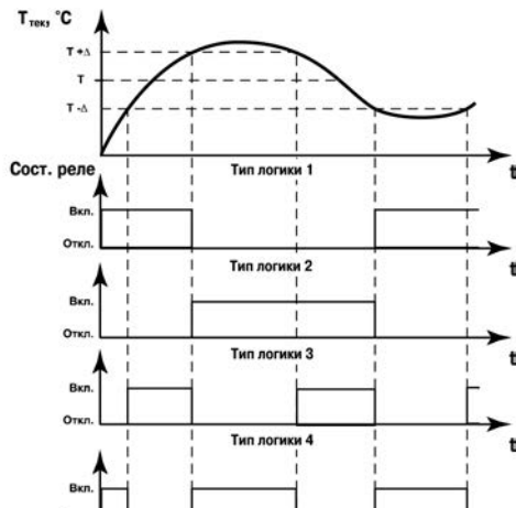
Рисунок 3.10 – Типы логики при работе ЛУ в режиме устройства сравнения
