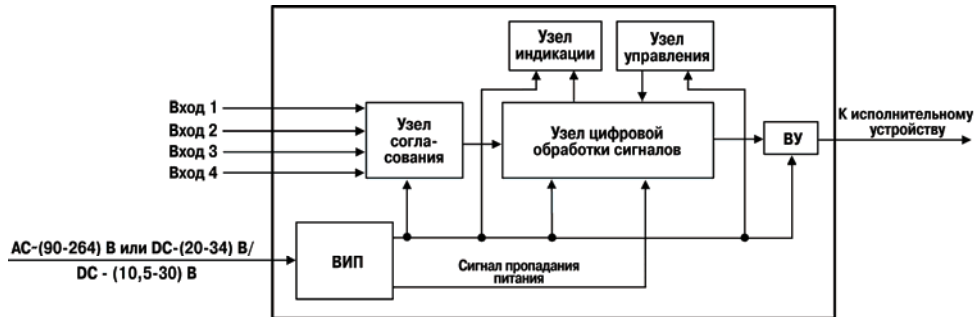
Рисунок 3.1 – Функциональная схема
