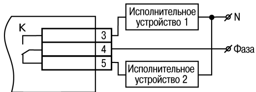
Рисунок Б.4 – Схема подключения нагрузки к ВУ типа Р
