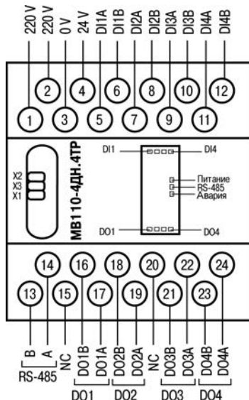
Рисунок Б.1 - Общий чертеж МК110
