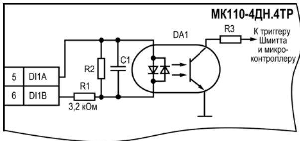
Рисунок Б.7 - Электрическая принципиальная схема дискретного входа МК110-220.4ДН.4ТР (схема других входов идентична приведенной)
