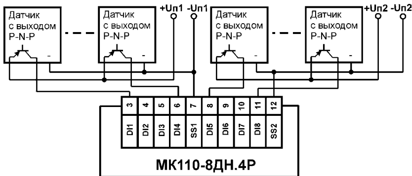
Рисунок Б.7 – Схема подключения к МК110-8ДН.4Р дискретных датчиков с транзисторным выходом р-п-п-типа
