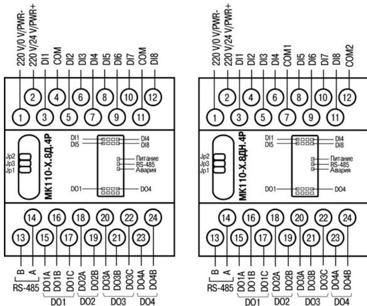
Рисунок Б.1 – Общий чертёж МК110
