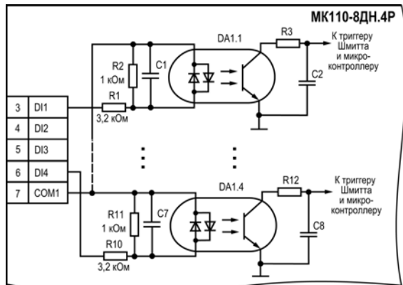
Рисунок Б.9 – Электрическая принципиальная схема группы дискретных входов МК110-8ДН.4Р (схема других групп входов идентична приведенной)
