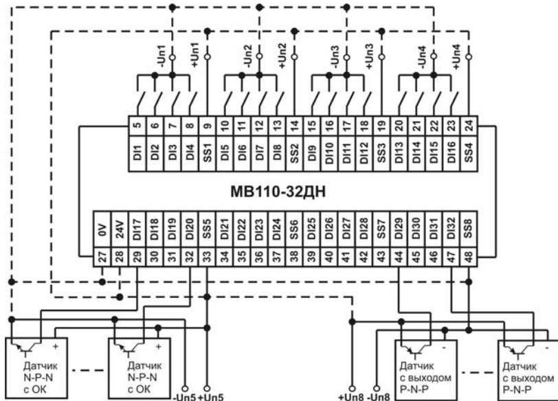
Рисунок Б.5 – Схема подключения к MB110-32DN дискретных датчиков с транзисторным выходом р-п-п-типа, п-п-п-типа с ОК и с выходом типа «сухой контакт» (пример)
