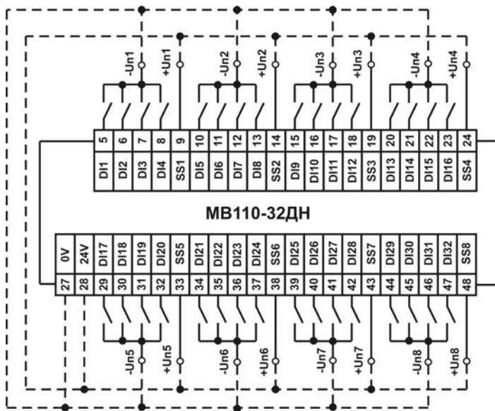
Рисунок Б.2 – Схема подключения к МВ110-32ДН дискретных датчиков с выходом типа «сухой контакт»
