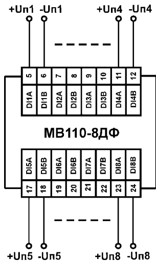
Рисунок Б.2 - Схема подключения к МВ110-8ДФ сигналов постоянного напряжения
