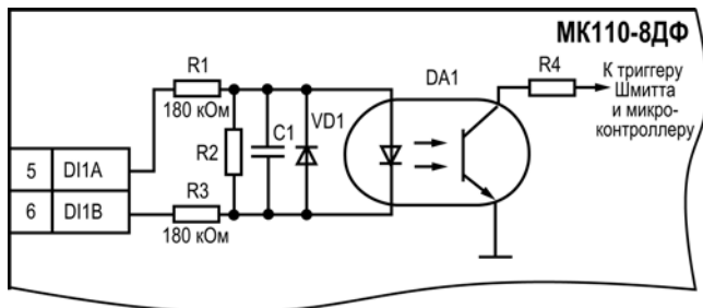
Рисунок Б.5 - Электрическая принципиальная схема входа МК110-8ДФ (схема других входов идентична приведенной)
