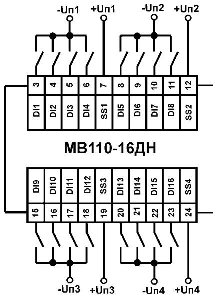
Рисунок Б.4 - Схема подключения к MB110-16DN дискретных датчиков с выходом типа «сухой контакт»
