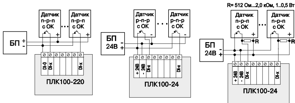
Рисунок Б.4 - Схемы подключения к ПЛК100 дискретных датчиков с полупроводниковым выходным каскадом: а – ПЛК100-220 датчик н-р-п-типа, б – ПЛК100-24 датчик р-н-р-типа, в – ПЛК100-24 датчик н-р-п-типа
