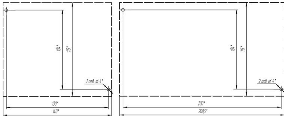
а) ПЛК110.X.30(32).X-X(M02)
