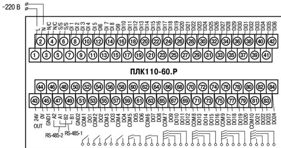
Рисунок Б.1 – Схема расположения и назначение клемм на ПЛК110-220.60.P(M02). Схема для ПЛК110-24.60.P(M02) – аналогична, полярность при подключении клемм питания аналогична рисунку Б.2
