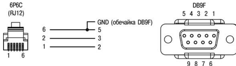
Рисунок Г.2 – Схема кабеля KC2
