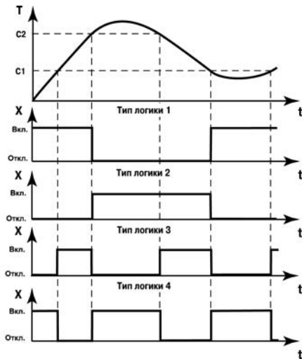
Рисунок 3.10 – Типы логики при работе устройства сравнения
