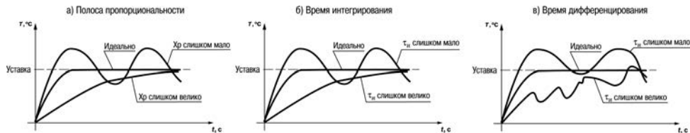
Рисунок 3.15 – Корректирование параметров регулирования
