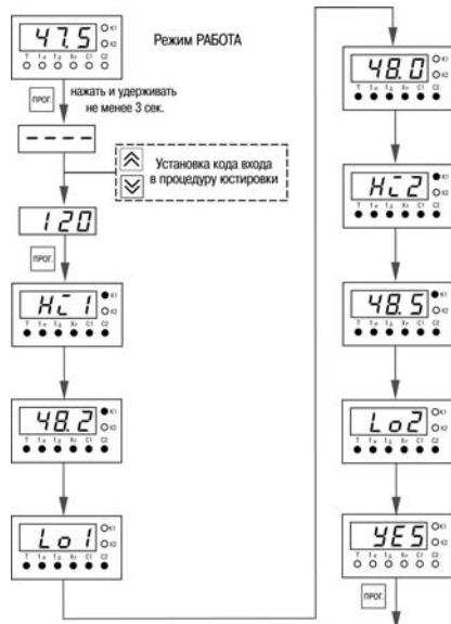
Рисунок Ж.2 – Последовательность запуска и индикации АНР для ТРМ10-Щ1.Р
