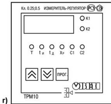
Рисунок 3.5 – Лицевая панель прибора для корпусов: а) настенного Н и щитового крепления Щ1; б) – щитового Щ2; в) – DIN-реечного Д; г) щитового Щ11
