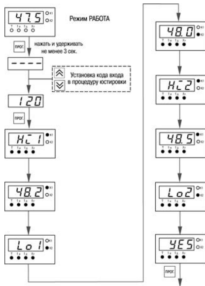
Рисунок Е.2 – Последовательность запуска и индикации АНР для ТРМ12-Щ1.Р
