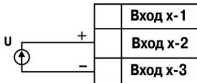
Рисунок Б.7 – Схема подключения активного датчика с выходом в виде напряжения -50...50 мВ или 0...1 В
