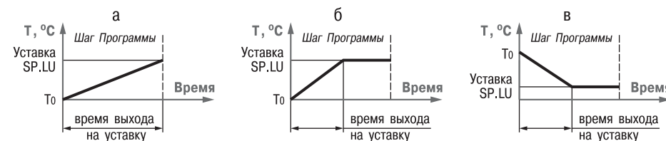
Рис. 10. Задание скорости выхода на Уставку
