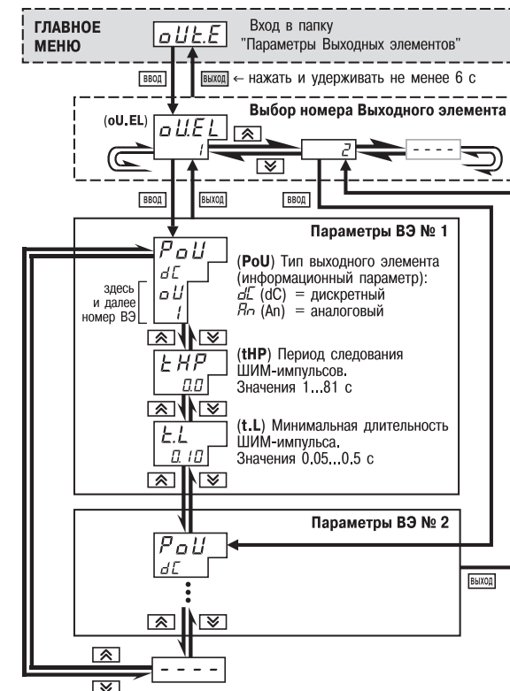
Рис. 46. Схема задания параметров Выходных элементов
