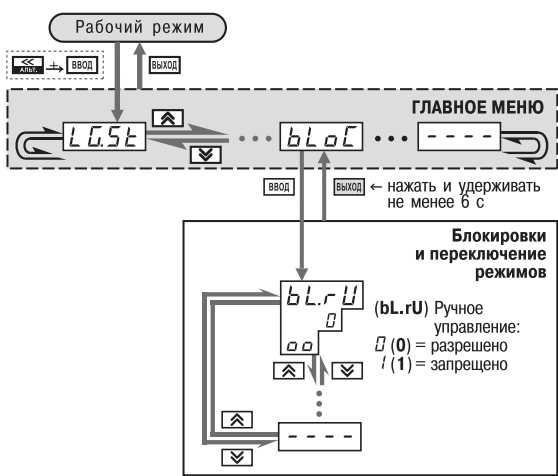
Рис. 53. Схема установки параметра блокировки ручного управления кнопками на лицевой панели прибора
