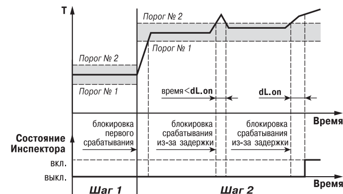
Рис. 8. Пример логики работы и блокировок срабатывания Инспектора
