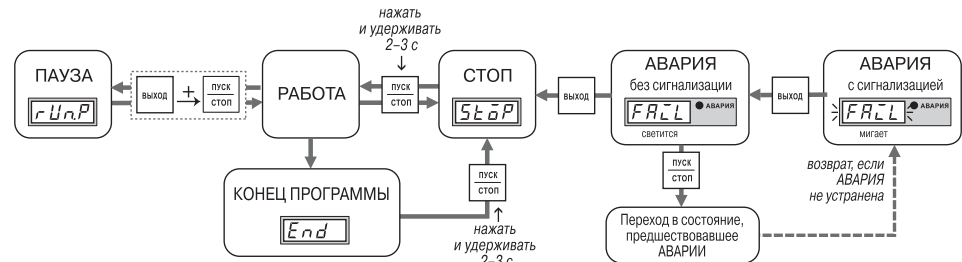
Рис. 12. Схема переключения состояний прибора
