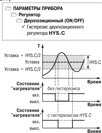
Рис. 7. Принцип работы Двухпозиционного регулятора
