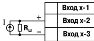
Рис. Б.12. Схема подключения активного датчика с токовым выходом 0 ... 5, 0 ... 20 или 4 ... 20 мА
