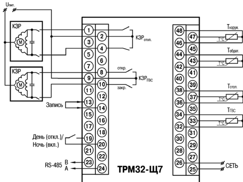
Рисунок В.3 – Схема подключения TPM32-Щ7
