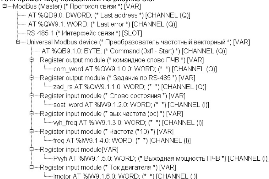
Рисунок 5.8 - Конфигурация ПЛК под задачу
