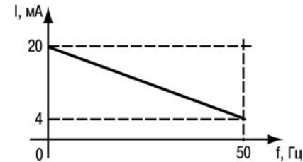
Рисунок 4.2 - Регулировочная характеристика ПЧВЗ
