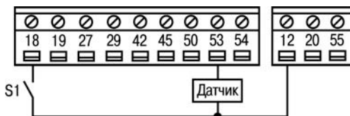
Рисунок 4.8 - Схема внешних подключений ПЧВЗ
