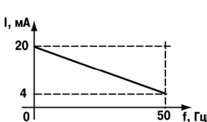
Рисунок 4.6 – Характеристика управления
