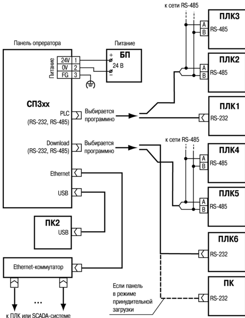
Рисунок Б.2 - Подключение панели к ПЛК и компьютерам (для конфигурирования) по различным интерфейсам
