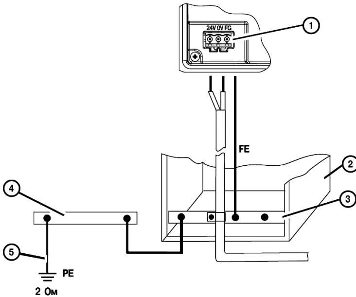
Рисунок Б.1 - Подключение выравнивающего потенциалы защитного заземления
