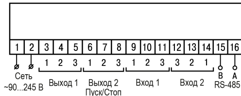
Рисунок 5.2 – Общая схема подключения TPM210-Н, -Щ1 и -Щ2
