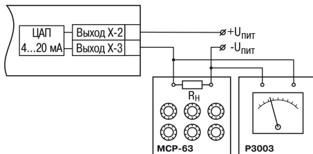
Рисунок 8.8 – Подключение ВУ1 типа У
