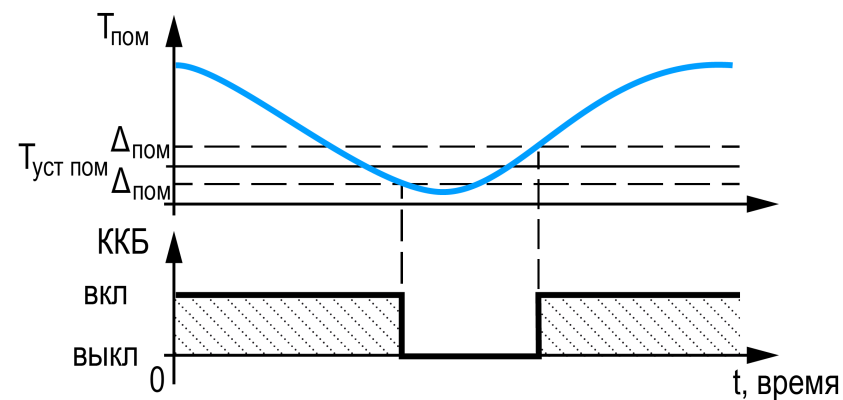
Рисунок 5.9 – Управление ККБ
