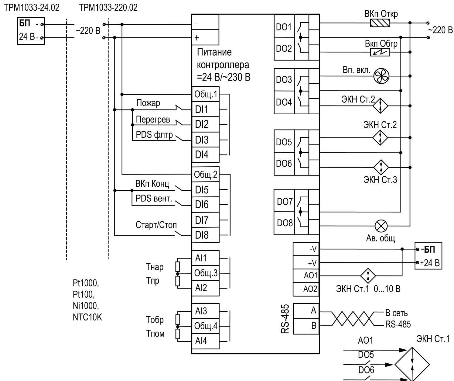
Рисунок 11.2 – Схема подключения Алгоритм 02 (Система с электрическим калорифером нагрева)
