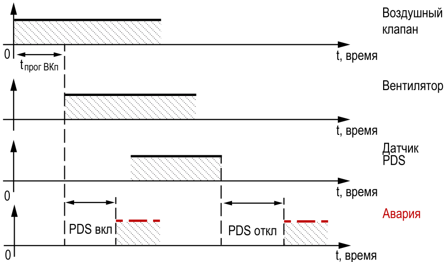
Рисунок 5.3 – Управление вентилятором притока
