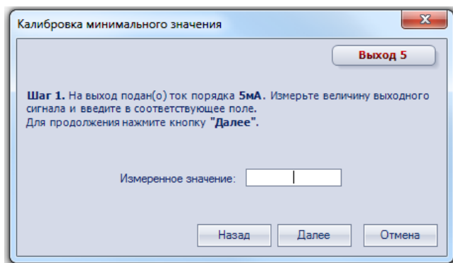
Рисунок 8.6 – Калибровка минимального значения
