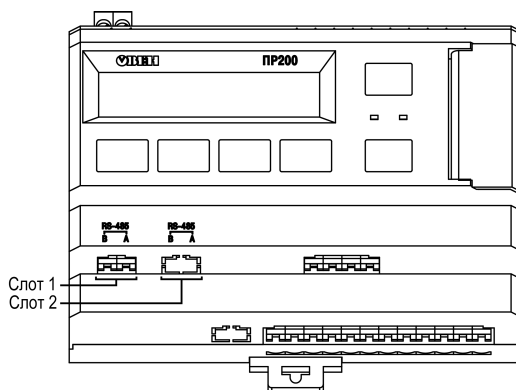
Рисунок 8.13 – Нумерация слотов RS-485
