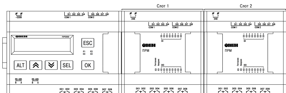
Рисунок 5.15 – Расположение модулей расширения на шине
