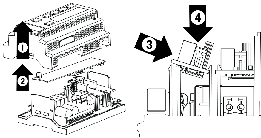
Рисунок 8.14 – Последовательность установки интерфейсной платы
