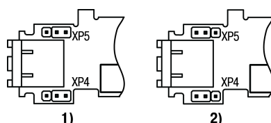
Рисунок 6.9 – Положение перемычек на плате ПР-ИП485: 1) подтягивающие резисторы подключены, 2) подтягивающие резисторы отключены
