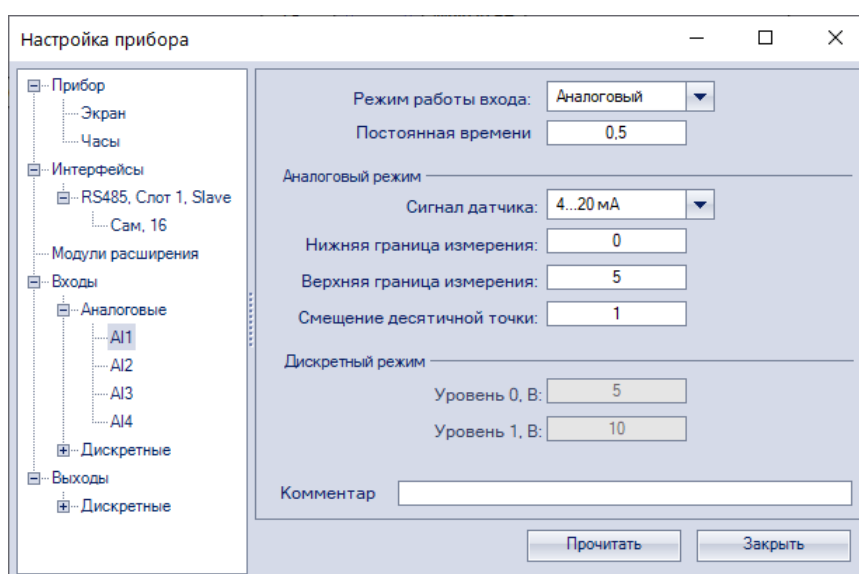
Рисунок 6.1 – Меню настройки прибора
