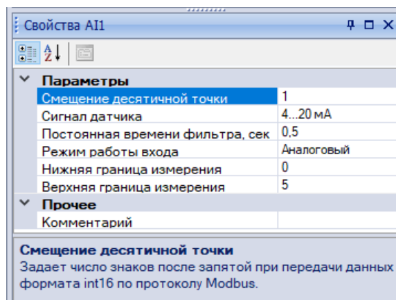
Рисунок 6.2 – Меню параметров
