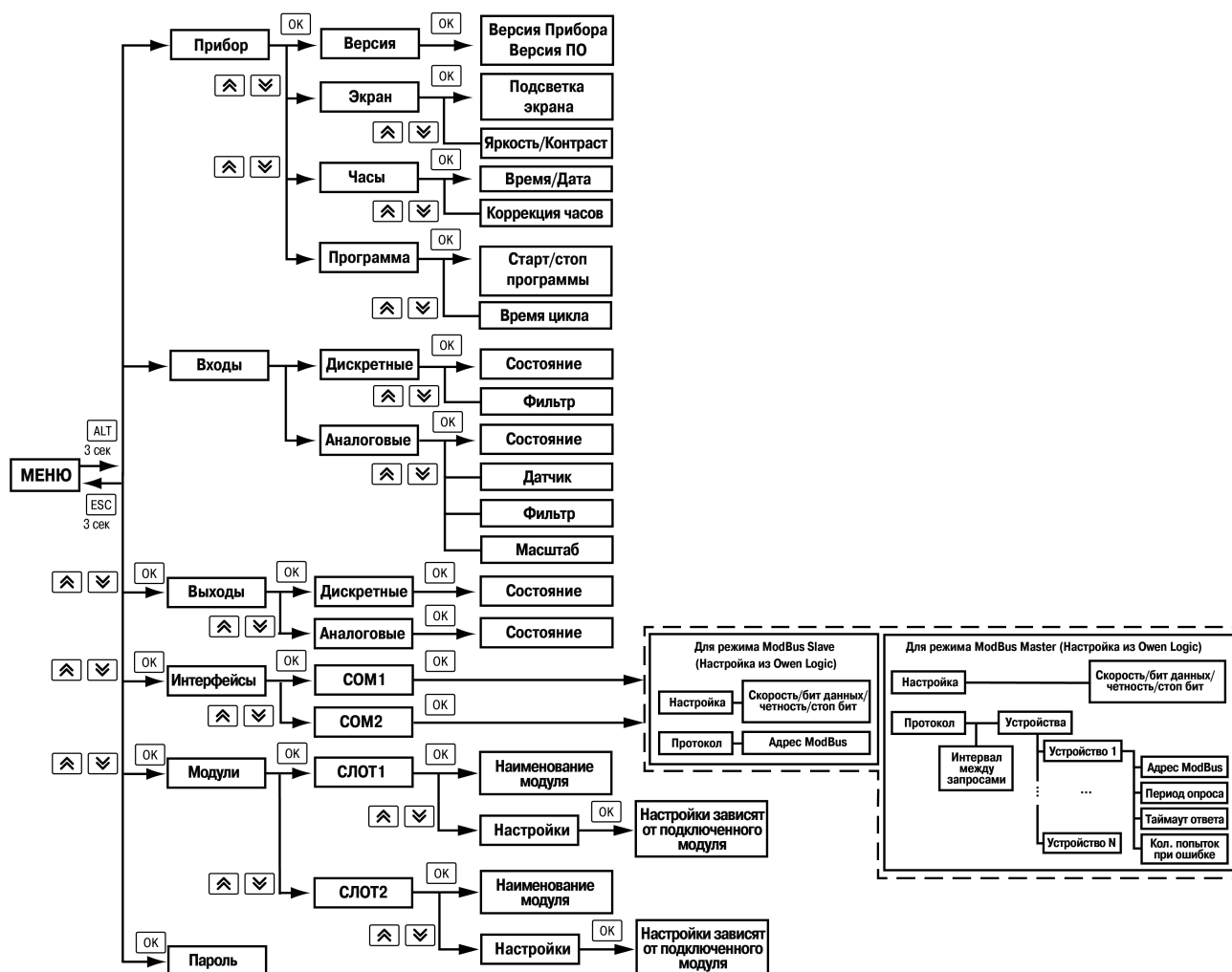
Рисунок 7.2 – Структура системного меню
