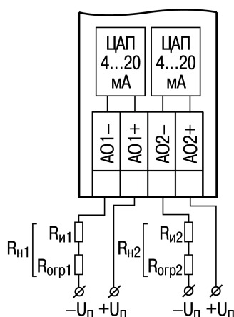
Рисунок 5.11 – Схема подключения нагрузки к ВЭ типа «И»
