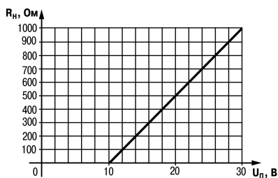
Рисунок 5.12 – График зависимости R_n ( U_n )
