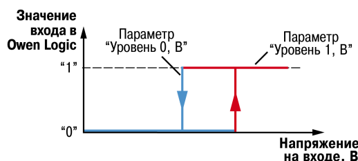
Рисунок 6.6 – Работа универсального входа в дискретном режиме
