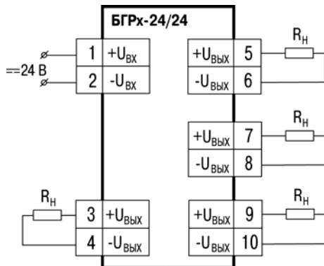
Рисунок 5.1 – Схема подключения
