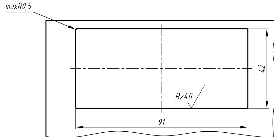
Посадочное место на щите
