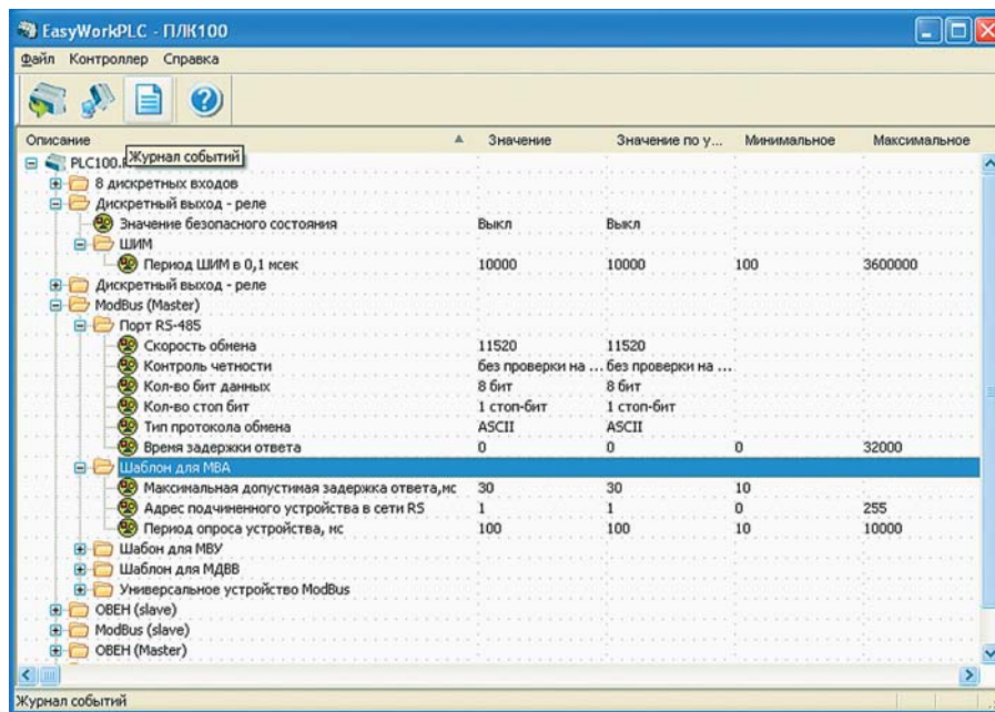
Рис. 2. Настроечные параметры периферийного оборудования программы EasyWorkPLC
