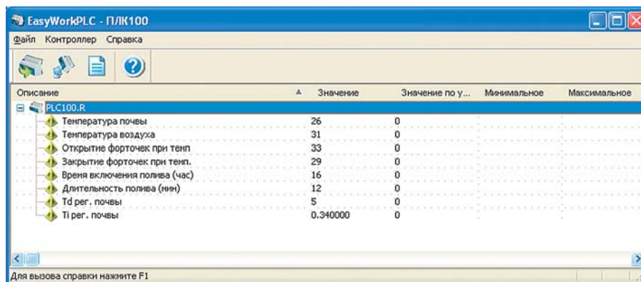
Рис. 1. Окно программы EasyWorkPLC с настройками коэффициентов и уставок
