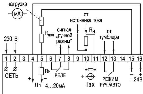
Рисунок Б.1 - Подключение УЗС1.х.И
