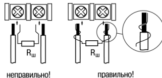
Рисунок 4.5 – подключение шунтирующего резистора
