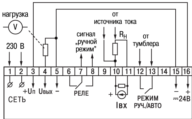
Рисунок Б.2 - Подключение УЗС1.х.У
