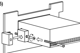
Рисунок 4.2 – Монтаж прибора щитового крепления
