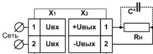
Рисунок 5.1 – Типовая схема подключения блока питания БП02Б – Д1 – 24
