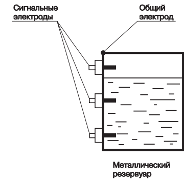
Рис. Б.2. Горизонтальное размещение в закрытом металлическом резервуаре
