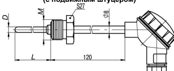
Рисунок А.9– Конструктивное исполнение 265 (с подвижным штуцером)
