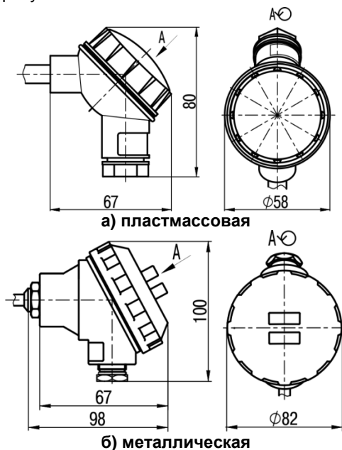
Рисунок Б.1 – Конструктивные исполнения коммутационных головок для ДТС-И и ДТП-И
