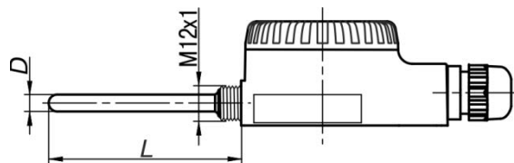
Рисунок А.10– Конструктивное исполнение 125
