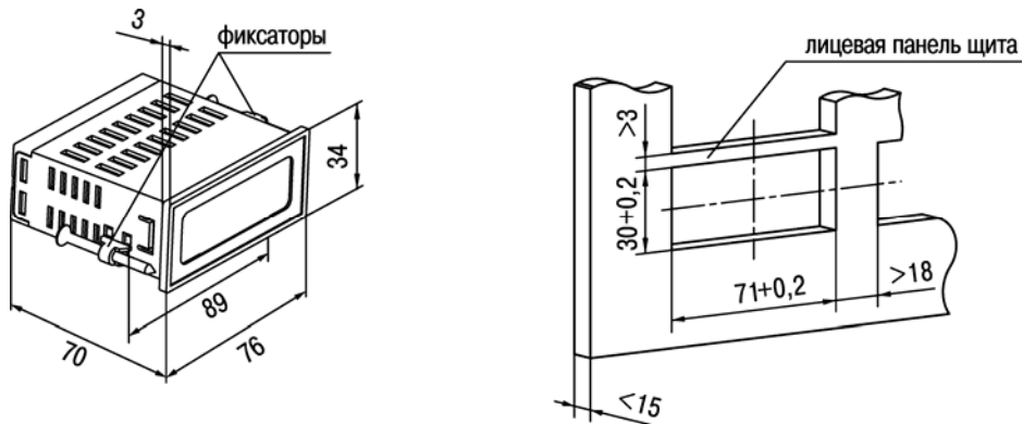
Рисунок А.1 – Габаритный чертеж прибора в корпусе ЩЗ
