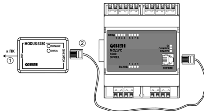
Рисунок Б.1 – Схема подключения Модус 5280 к Модус 5680
