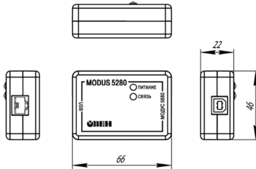
Рисунок А.1 – Габаритный чертеж прибора
