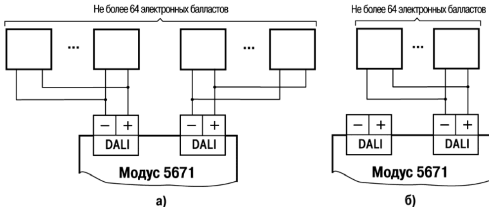
Рисунок Б.1 – Схемы подключения
