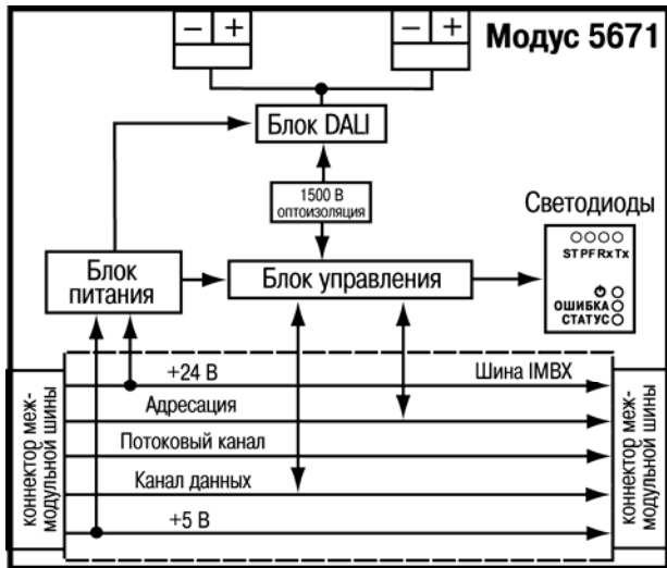
Рисунок 3.2 – Структурная схема модуля
