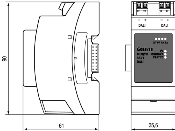
Рисунок А.1 – Габаритный чертеж
