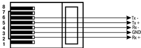
Рисунок Б.3 – Кабель связи ПЛК308 по RS-422 с внешним устройством
