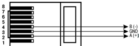
Рисунок Б.1 – Кабель связи ПЛК308 по RS-485 с внешним устройством
