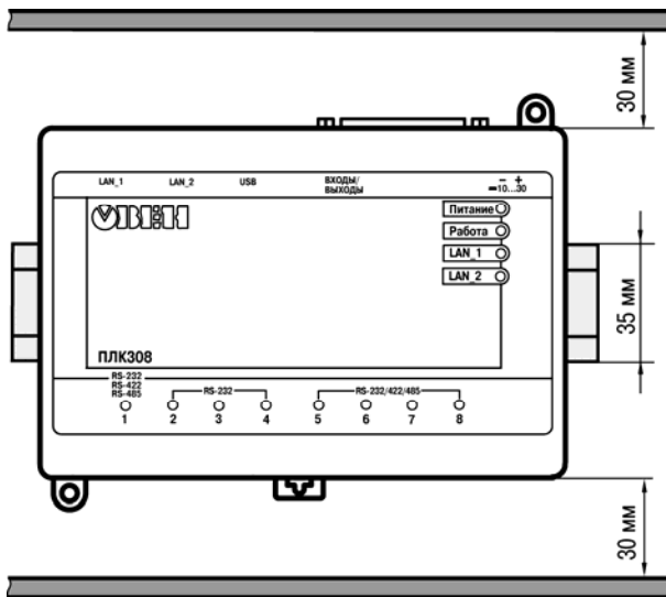
Рисунок А.3 – Расстояние до стенок корпуса ПЛК308 при монтаже для обеспечения вентиляции
