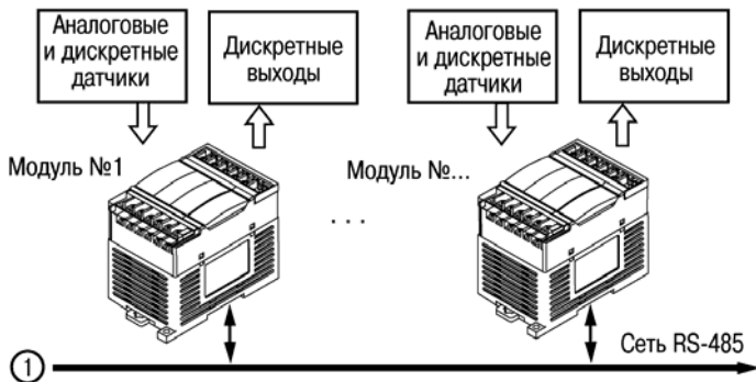
Рисунок 6.2 – Пример структуры соединений при использовании ПЛК308 в системе управления (продолжение)
