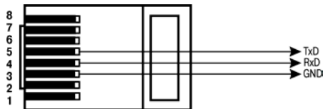
Рисунок Б.2 – Кабель связи ПЛК308 по RS-232 с внешним устройством
