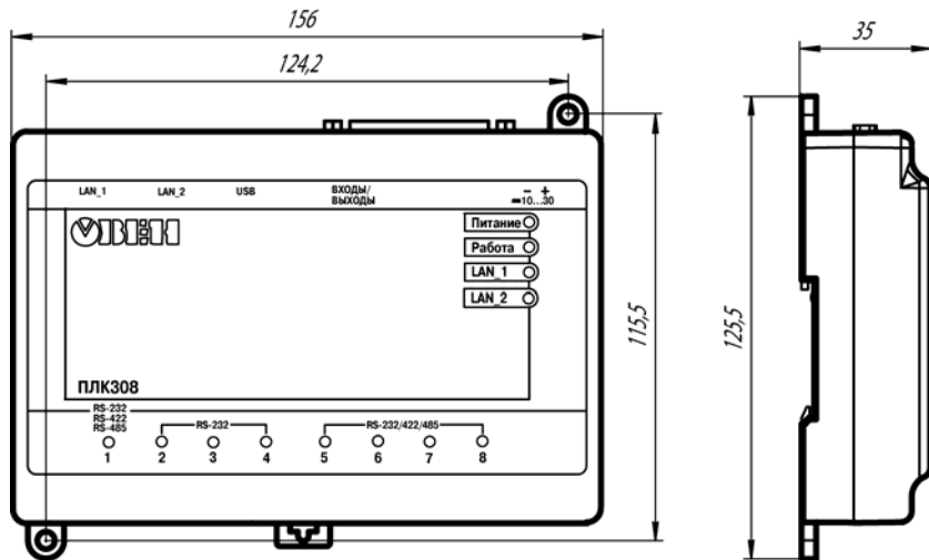
Рисунок А.1 – Габаритные размеры ПЛК308
