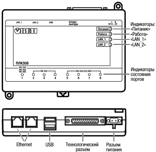
Рисунок 3.1 – Внешний вид ПЛК308
