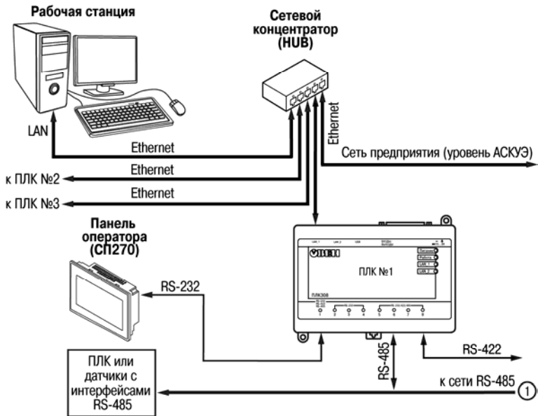
Рисунок 6.2 – Пример структуры соединений при использовании ПЛК308 в системе управления
