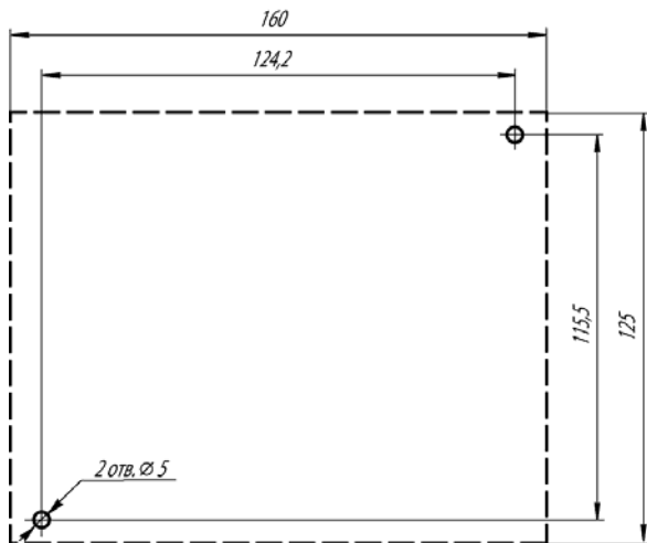
Рисунок А.2 – Разметка для установки на щит
