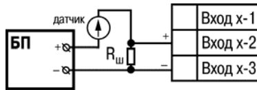
Рисунок Б.5 – Подключение активного датчика с токовым выходом 0...5 \text{ мА} или 0(4)...20 \text{ мА} ( R_{ш} = 100,0 \text{ Ом} \pm 0,1\% )
