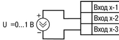
Рисунок Б.4 – Подключение активного датчика с выходом в виде напряжения 0...1 \text{ В}
