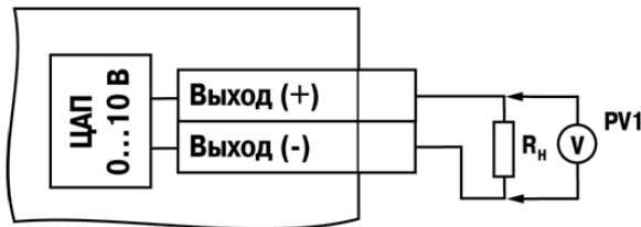
Рисунок Б.7 – Схема подключения нагрузки к ВЭ типа «У». R_{н} > 2 \text{ кОм}
