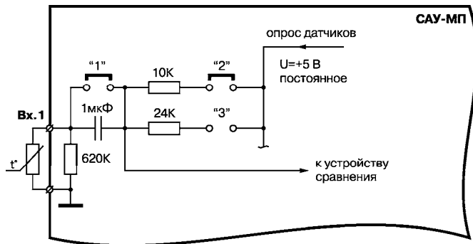
Рисунок 3.8 - Подключение термисторов и позисторов
