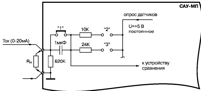
Рисунок 3.7 - Подключение датчиков с унифицированным сигналом
