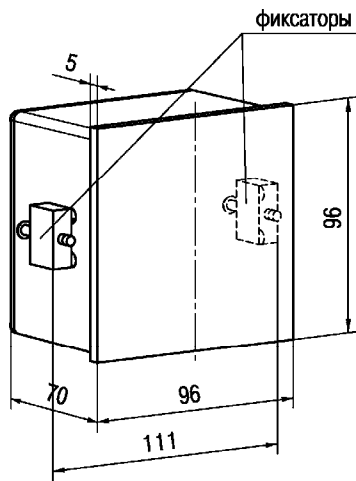
Рисунок А.2 - Корпус щитового крепления типа Щ1
