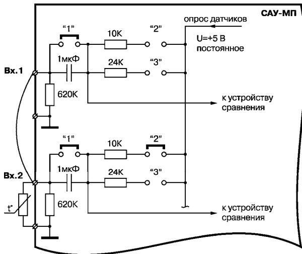
Рисунок 3.9 - Параллельное подключение датчика температуры к двум разным входам
