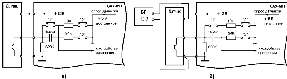
Рисунок 3.5 - Схема подключения емкостных выключателей: а) питание от прибора, б) питание от внешнего источника
