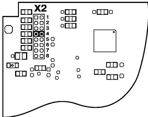
Рисунок 6.1 - Положение перемычки на плате индикации в режиме измерения напряжения на входах
