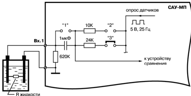
Рисунок 3.4 - Схема подключения кондуктометрического зонда (с расположением переключек)
