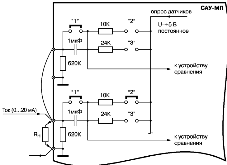
Рисунок 3.10 - Параллельное подключение датчика с нормирующим преобразователем
