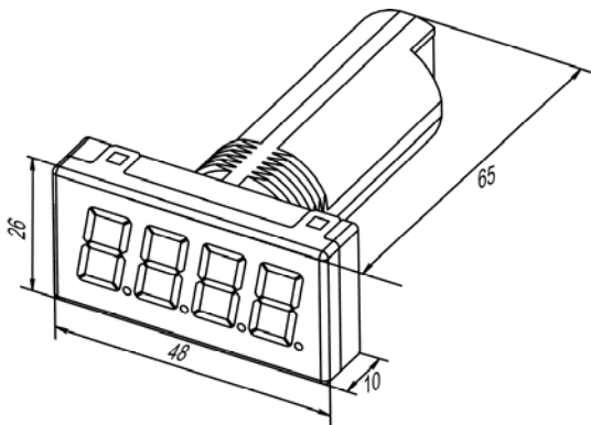
Рисунок А.1 – Габаритный чертеж корпуса прибора
