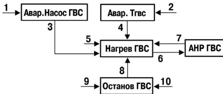
Рисунок 4.1 – Схема перехода между режимами контура ГВС
