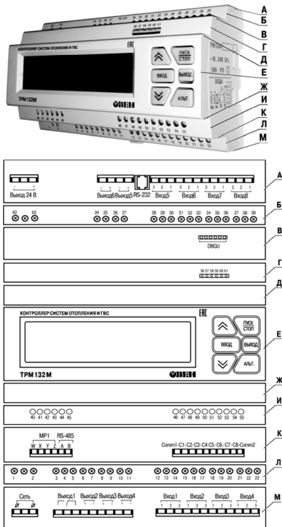
Рисунок 3.1 – Прибор ТРМ132М-01: клеммники, элементы индикации и управления
