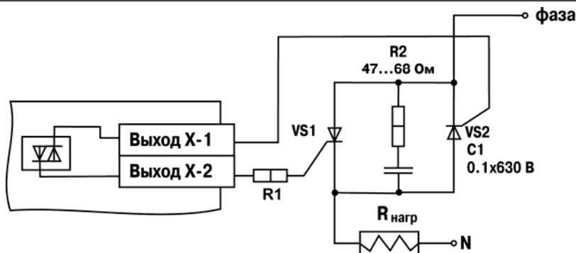
Рисунок Б.11 – Схема подключения нагрузки к ВУ типа С двух тиристорных, подключенных встречно-параллельно
