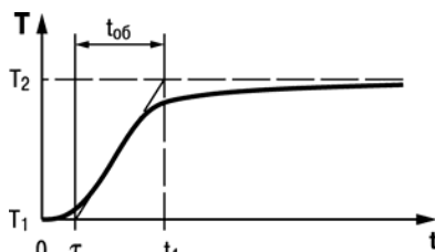
Рисунок Г.2 – График переходной функции
