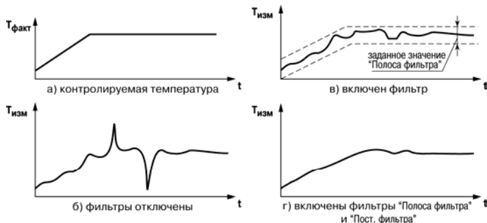
Рисунок 3.3 – Временные диаграммы работы цифровых фильтров показаний датчика
