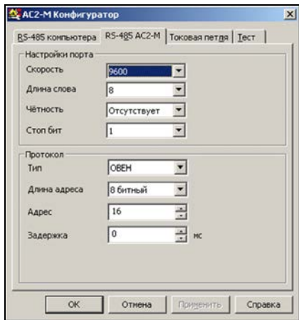
Рисунок Е.2 – Конфигуратор AC2-M.
