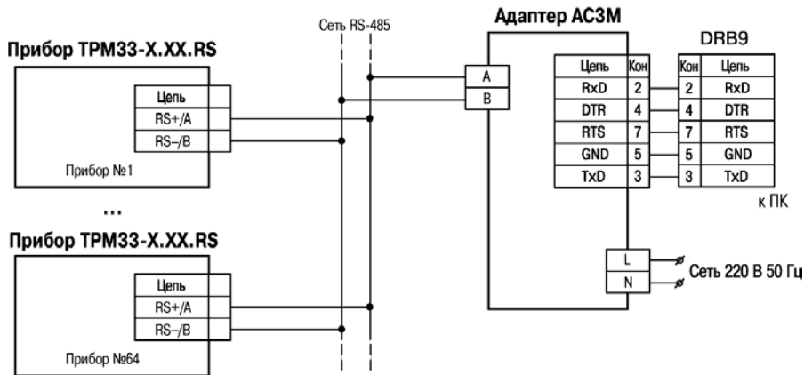
Рисунок В.4 – Схема подключения TPM33-X.X.RS к адаптеру сети АС3М
