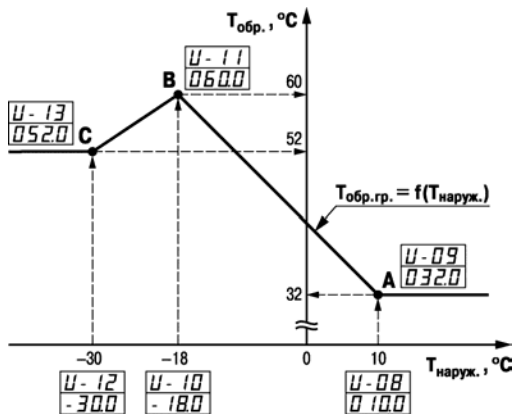
Рисунок Г.1 – Пример графика T_{\text{обгр.гр.}} = f(T_{\text{наруж.}}) (параметры для ТРМ33-Щ4)
