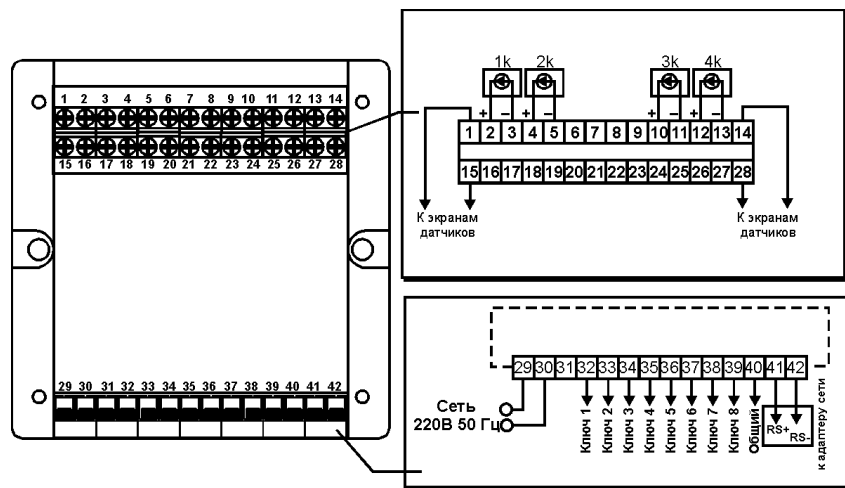
Схема подключения прибора TRM34 при использовании в качестве датчиков источников унифицированных токов или напряжений
